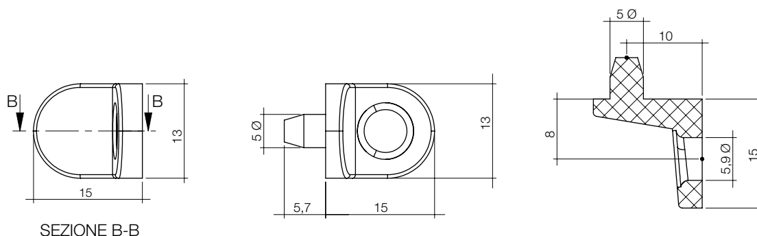
SEZIONE B-B
