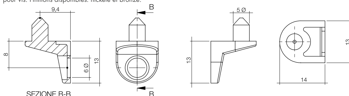
SEZIONE B-B
